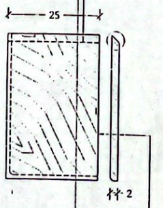
PLANK D4 DETAIL تایخچه چوبی شماره ۴
