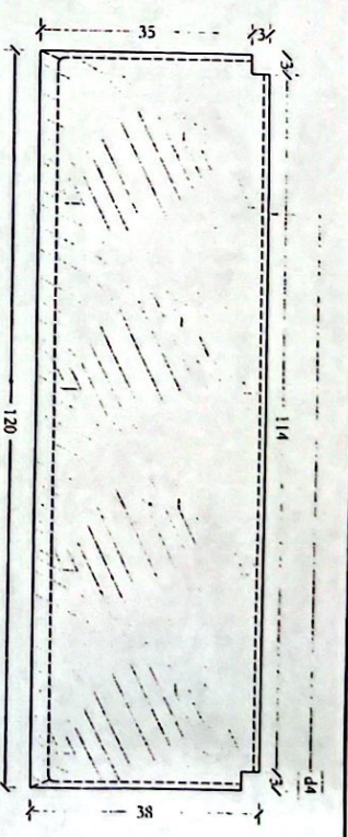
PLANK D4 DETAIL تایخچه چوبی شماره ۴
